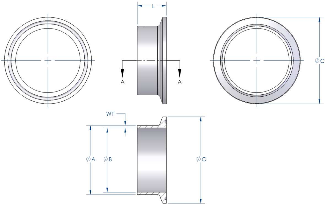
FERRULES - DIN 32676 - SERIES 1
