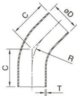
DIN 45 Deg Long Leg
