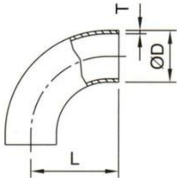
DIN 90 Deg Short Leg
