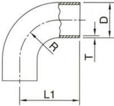
DIN 90 Deg Short Leg
