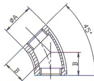
Elbow 45°
